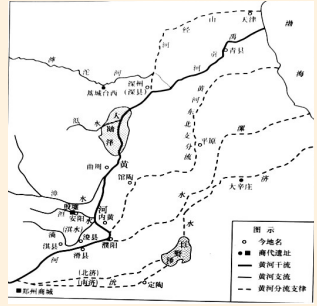
商代黄河下游河道形势图
